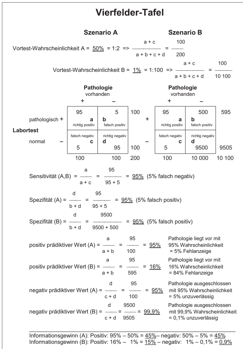
Abbildung 2: die Vierfelder-Tafel.
