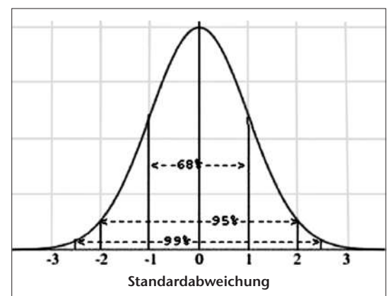
Abbildung 1: Gauss'sche Normalverteilung.
